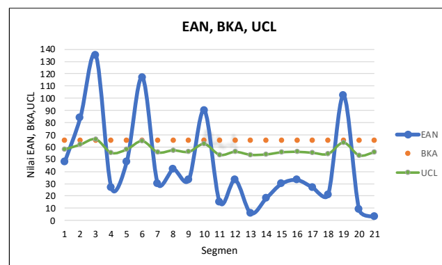
Gambar 7. Nilai Equivalent Accident Number (EAN), Batas Kontrol Atas (BKA), dan Upper Control Limit (UCL) pada setiap segmen di jalan Lintas Tengah Sumatera Km 14-Km 34
